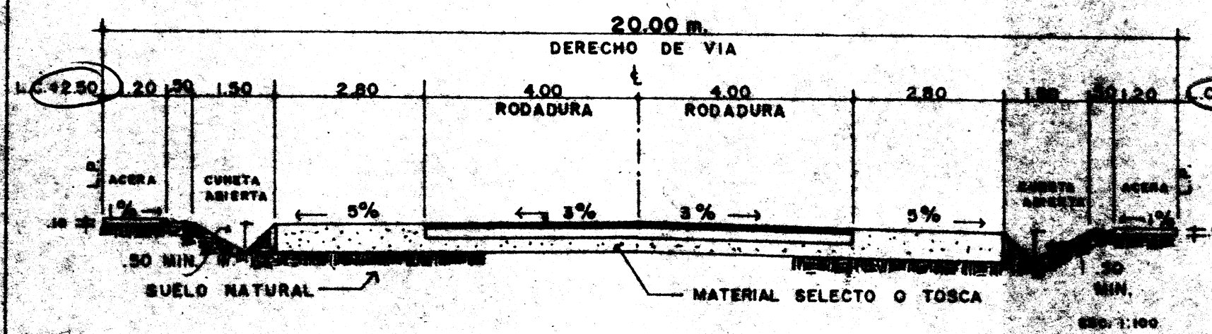
CARRETERA INTERAMERICANA RODADURA DE HORMIGON
