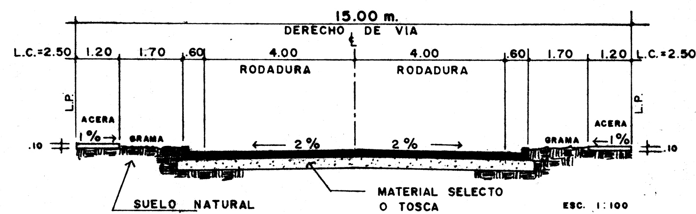
VIA SECUNDARIA A RODADURA DE HORMIGON
