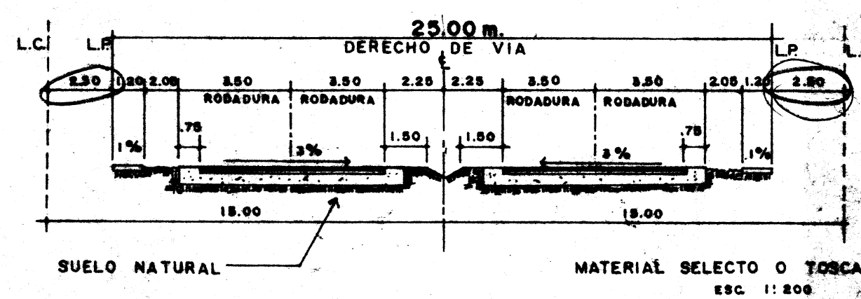
VIA INTER-URBANA C RODADURA DE ASFALTO
