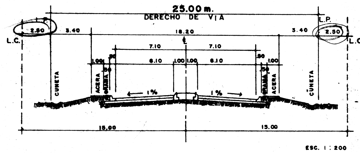
VIA INTER-URBANA A RODADURA DE HORMIGON
