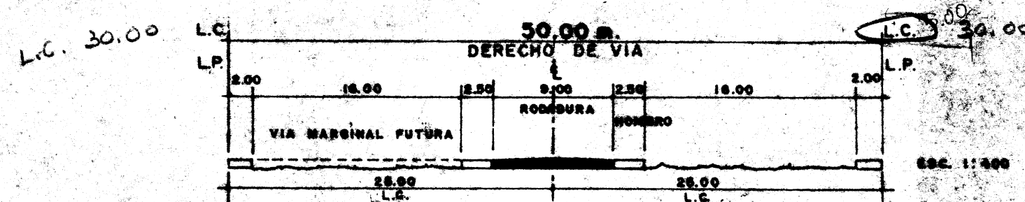
CARRETERA INTERAMERICANA RODADURA DE HORMIGON
