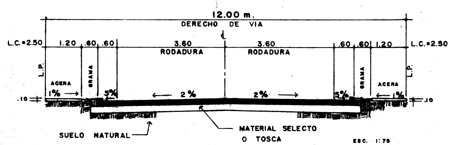
VIA COLECTORA A RODADURA DE HORMIGON
