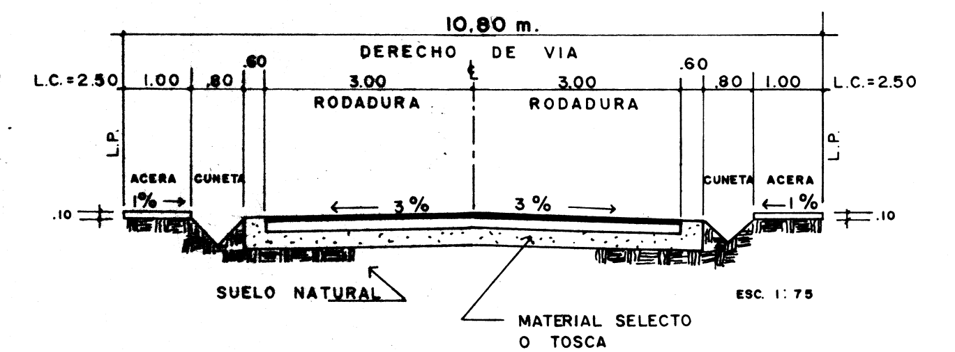
VIAS LOCALES RODADURA DE ASFALTO
