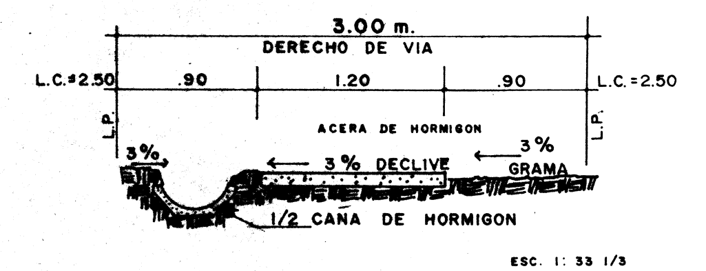
CALLE SIN SALIDA
