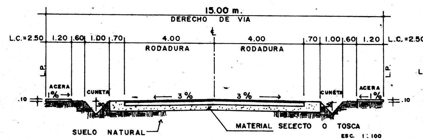
VIA SECUNDARIA B RODADURA DE ASFALTO
