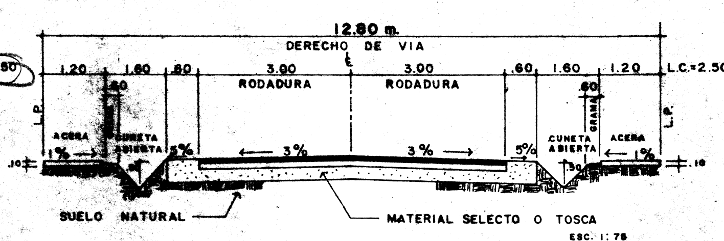
VIA COLECTORA B RODADURA DE ASFALTO
