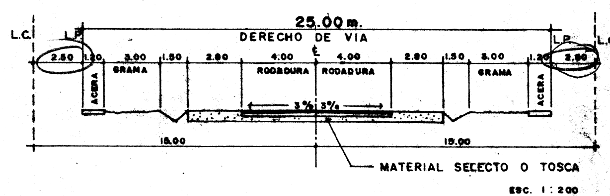
VIA INTER-URBANA B RODADURA DE ASFALTO
