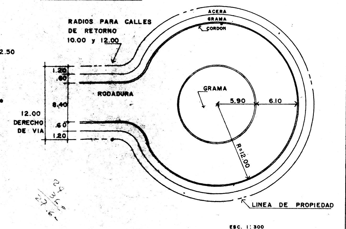
CALLE SIN SALIDA
