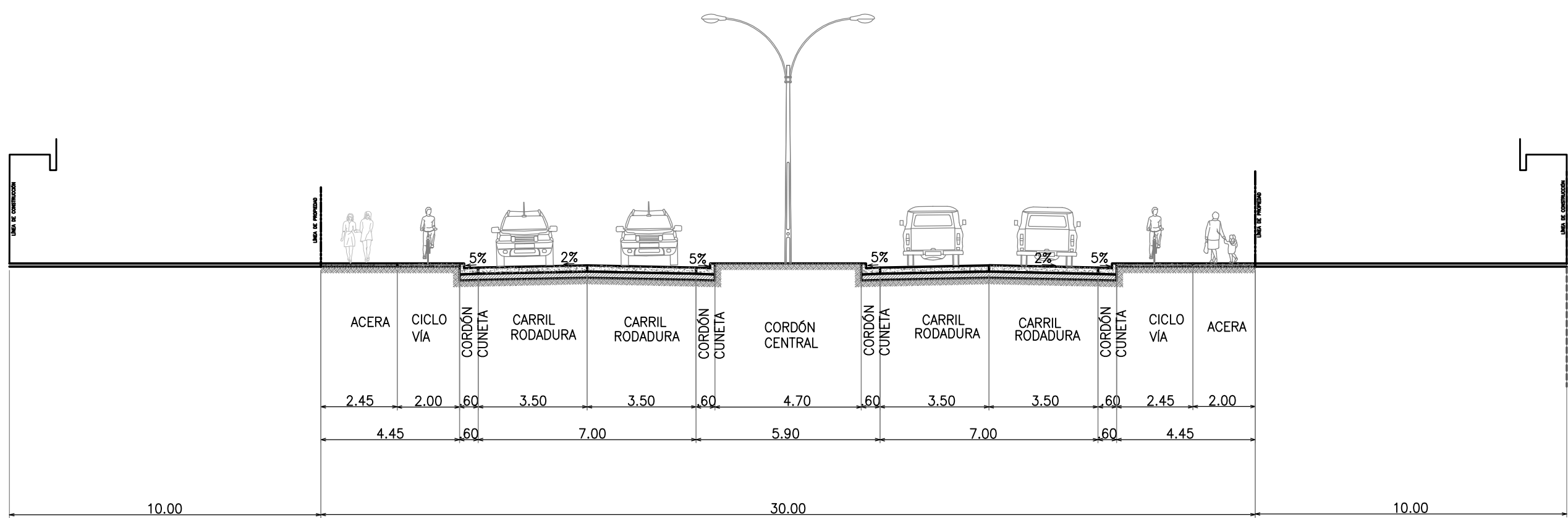
SECCIÓN DE VÍA DE 30.00 TÍPICA ESC.: 1 : 150
