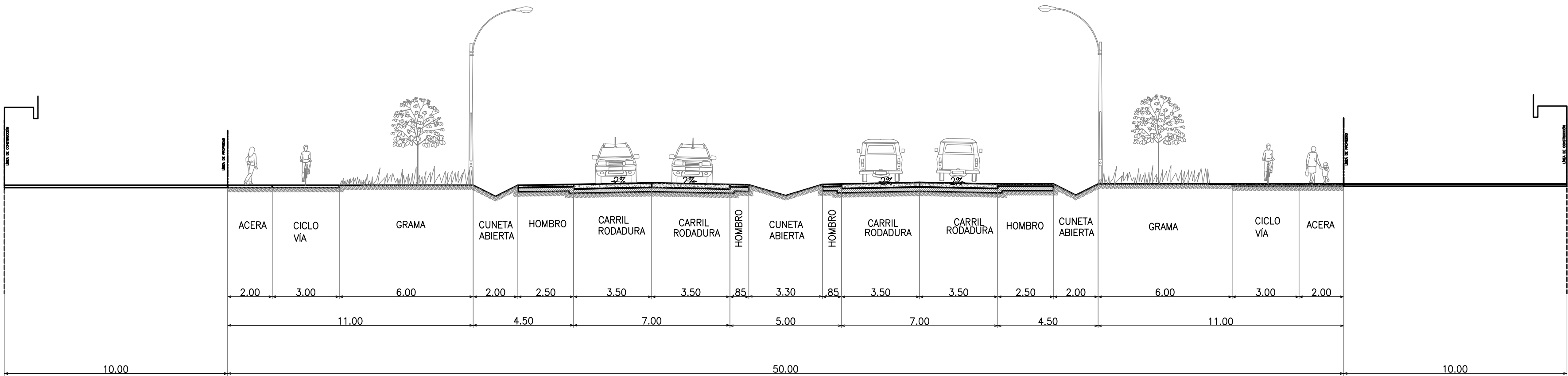
SECCIÓN DE VÍA DE 50.00 TÍPICA ESC.: 1 : 150
