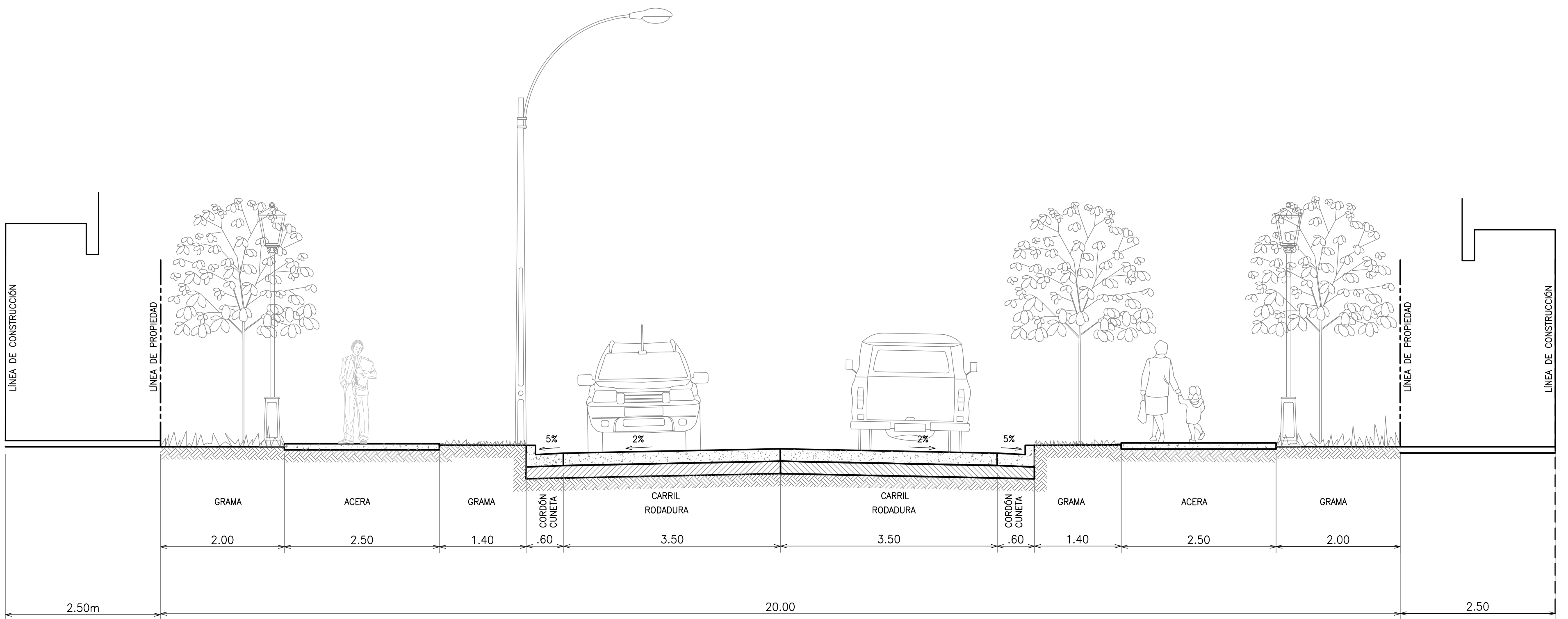
SECCIÓN DE VÍA DE 20.00 TÍPICA A ESC.: 1 : 50
