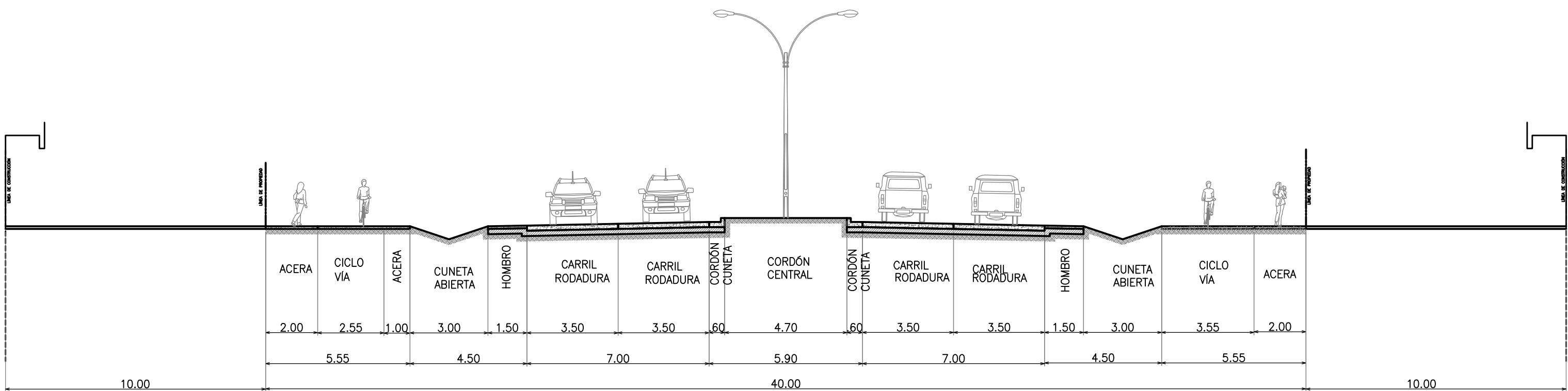
SECCIÓN DE VÍA DE 40.00 TÍPICA ESC.: 1 : 150
